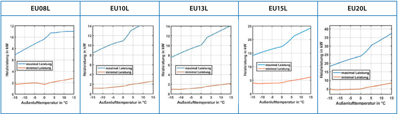
Leistungsdiagramme bei 5K Spreizung (35°C Vorlauftemperatur)
